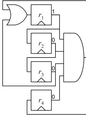
Figure 2.9: Exemple de circuit séquentiel
