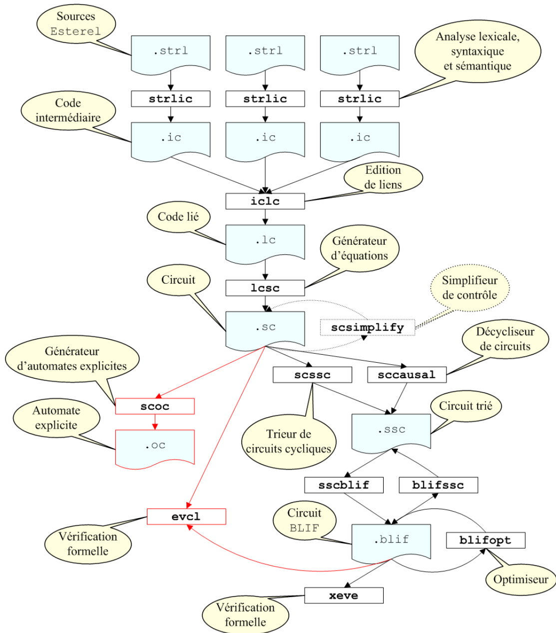
Figure 2.6: La chaîne de compilation d'Esterel v5_9x
