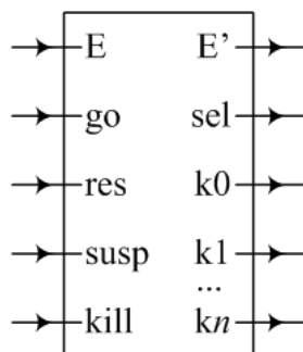
Figure 2.3: Bloc de base des circuits Esterel
