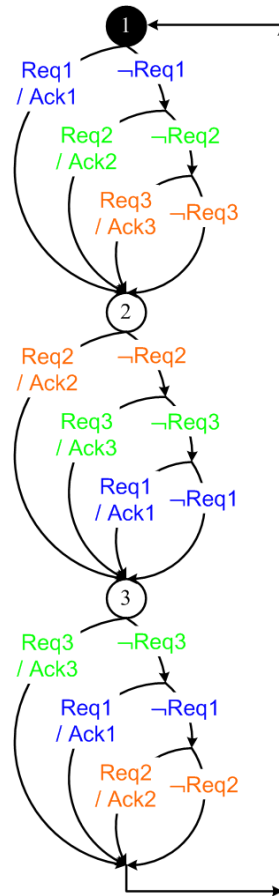
Figure 4.4: Automate de l'arbitre de bus (à 3 cellules)
