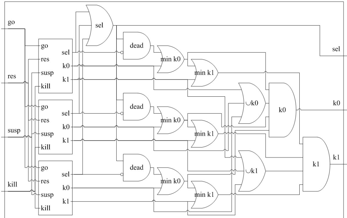
Figure 3.6: Circuit généré pour les constructions parallèles (3 composants)
