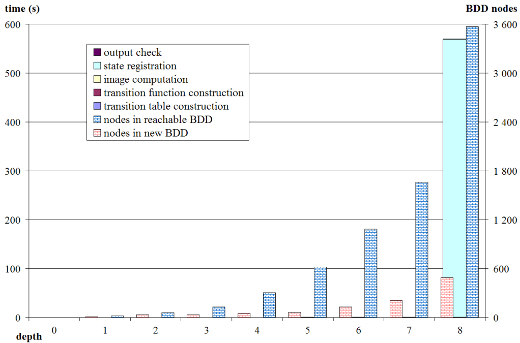
Figure 6.2: TI : temps et nœuds de BDDs par profondeur
