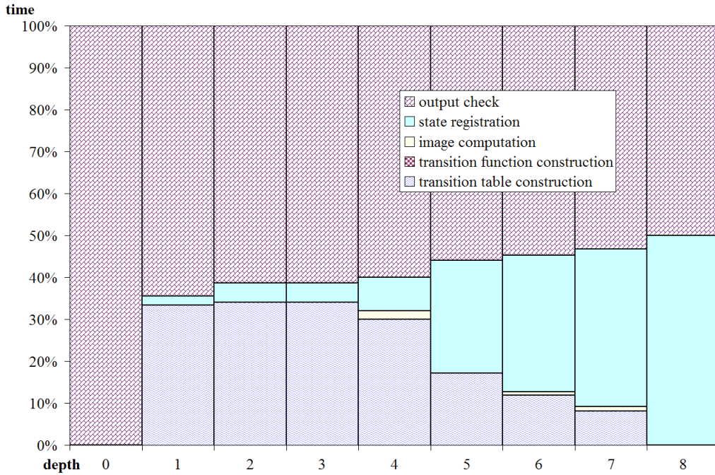
Figure 6.3: TI : distribution du temps par profondeur
