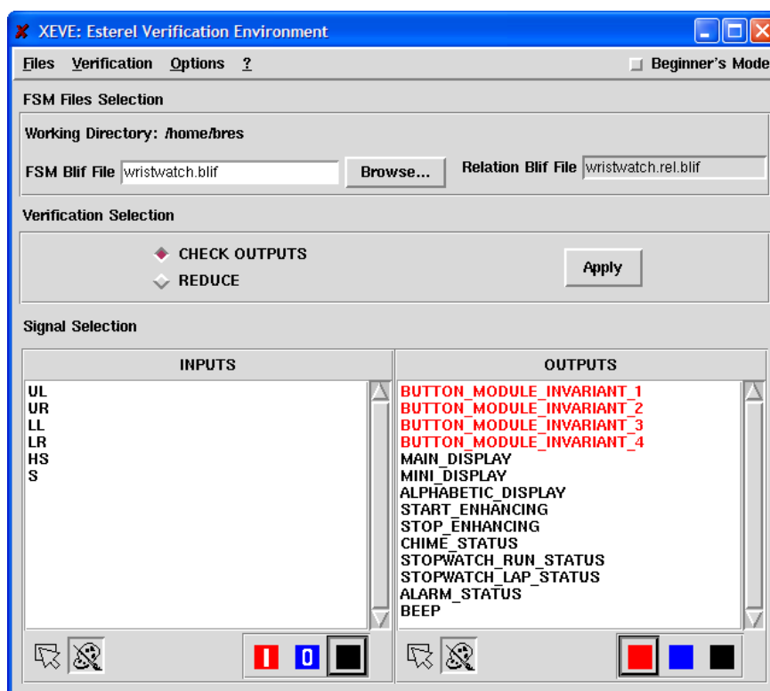
Figure 3.1: L’interface graphique Xeve
