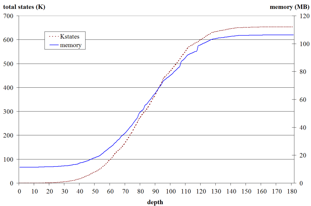
Figure 6.6: TI : progression des états totaux et du temps d'analyse avec la profondeur
