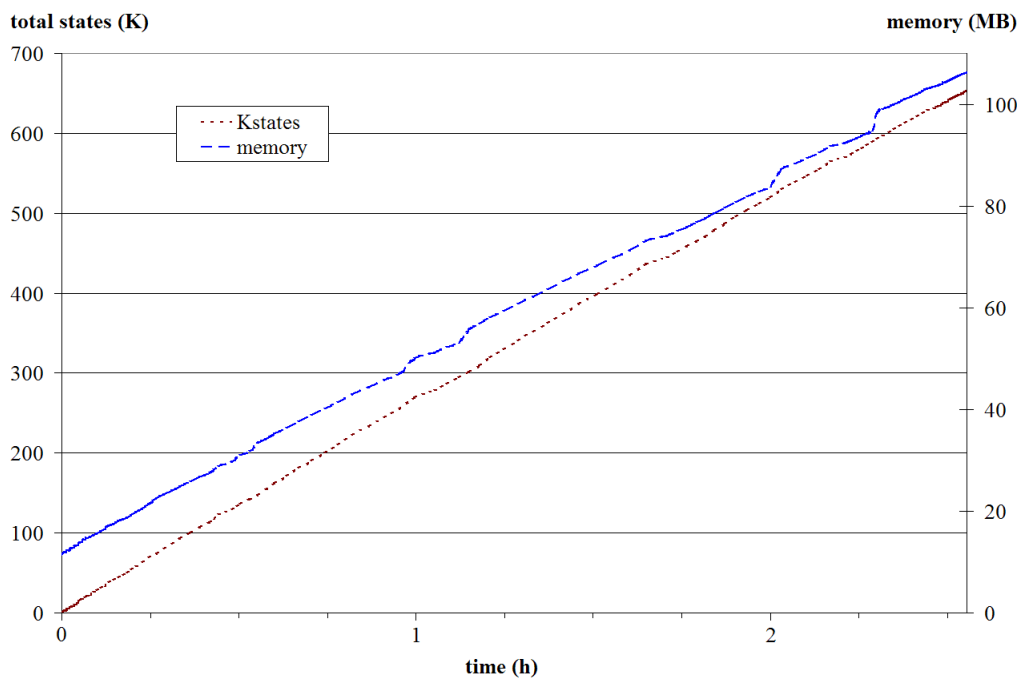
Figure 6.7: TI : progression des états analysés et de la consommation mémoire avec le temps
