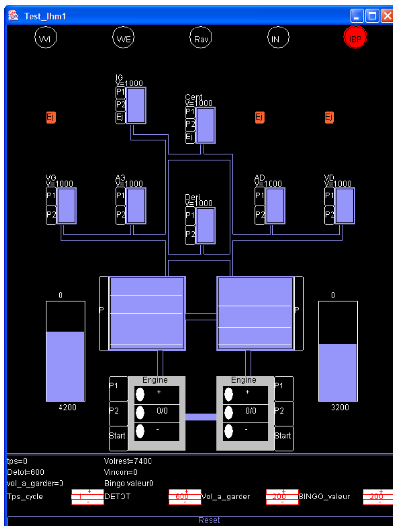
Figure 6.1: Interface graphique de l'application Carburant
