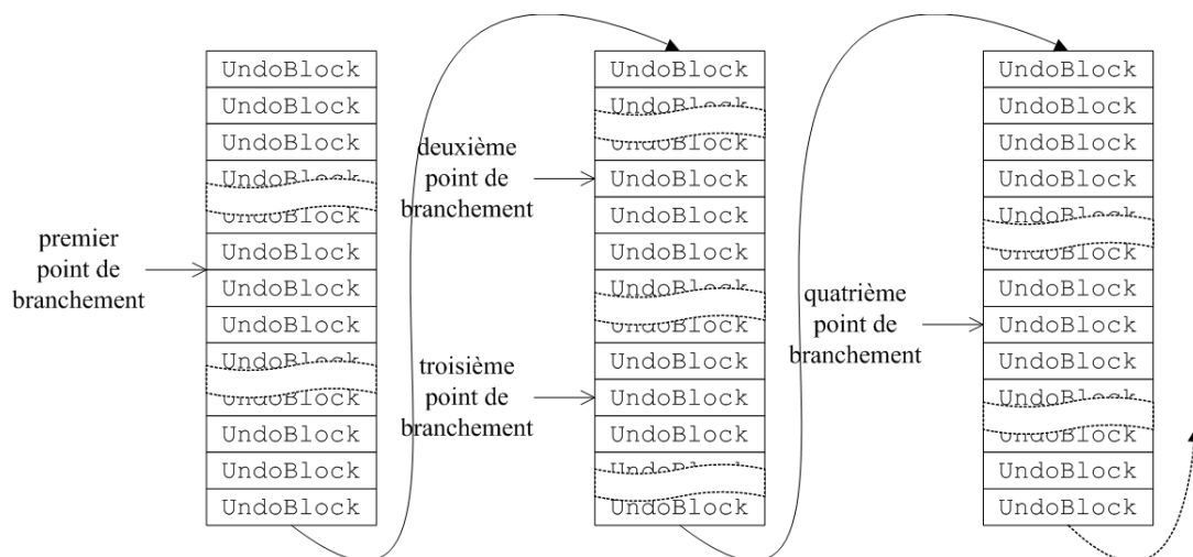
Figure 4.9: Chaînage des piles d'UndoBlocks
