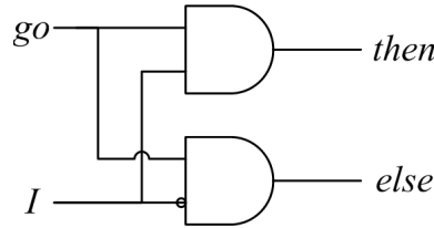
Figure 3.3: Fragment de circuit généré par l'expression present I then ... else ...
