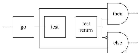
Figure 4.8: Sous-circuit correspondant à une instruction de test
