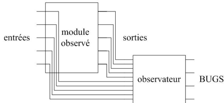
Figure 2.10: Observateur exécuté en parallèle du modèle à observer
