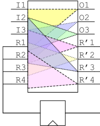
Figure 3.2: Cône d'influence des fonctions d'un circuit
