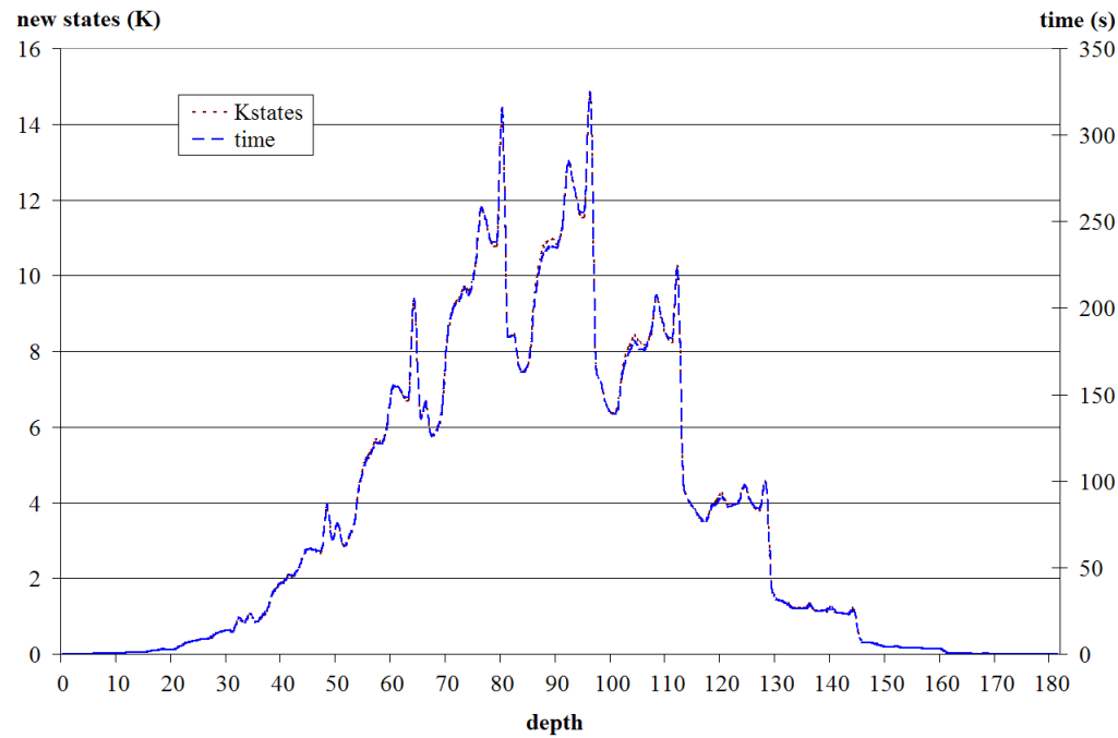
Figure 6.5: TI : nouveaux états découverts et temps d'analyse par profondeur
