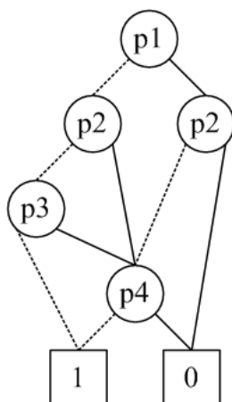
Figure 3.7: BDD de l'arbre de sélection du Programme 2.6
