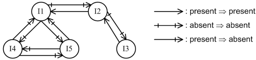
Figure 4.1: Graphe de relations entre entrées
