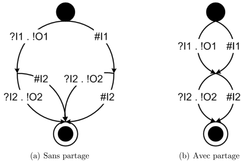
Figure 4.10: Automates avec et sans partage du programme Esterel 4.4
