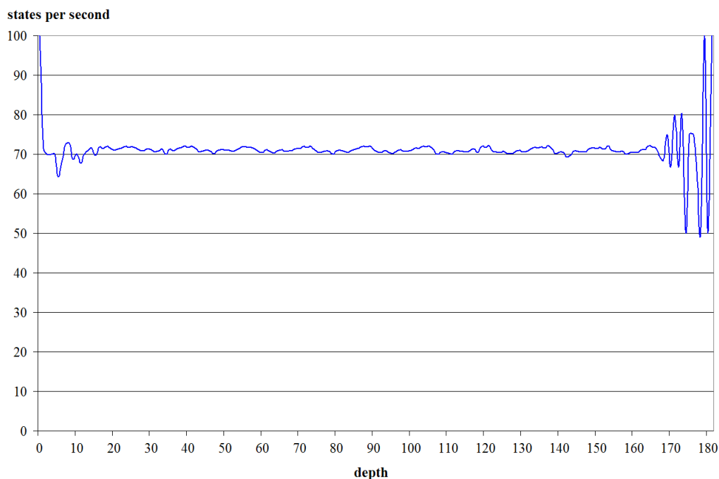
Figure 6.8: TI : débit d'analyse des états par profondeur
