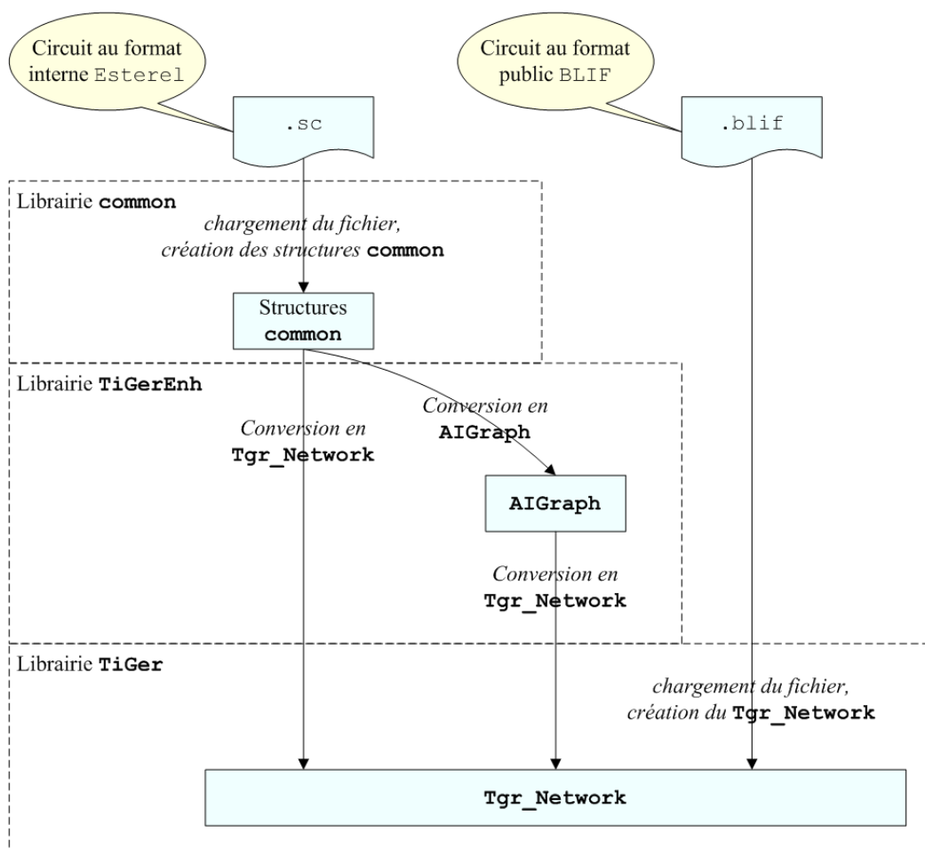
Figure 3.8: Flots de création de Tgr_Networks
