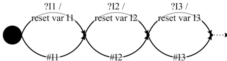
Figure 4.6: Début du graphe de transition d'initialisation de variables
