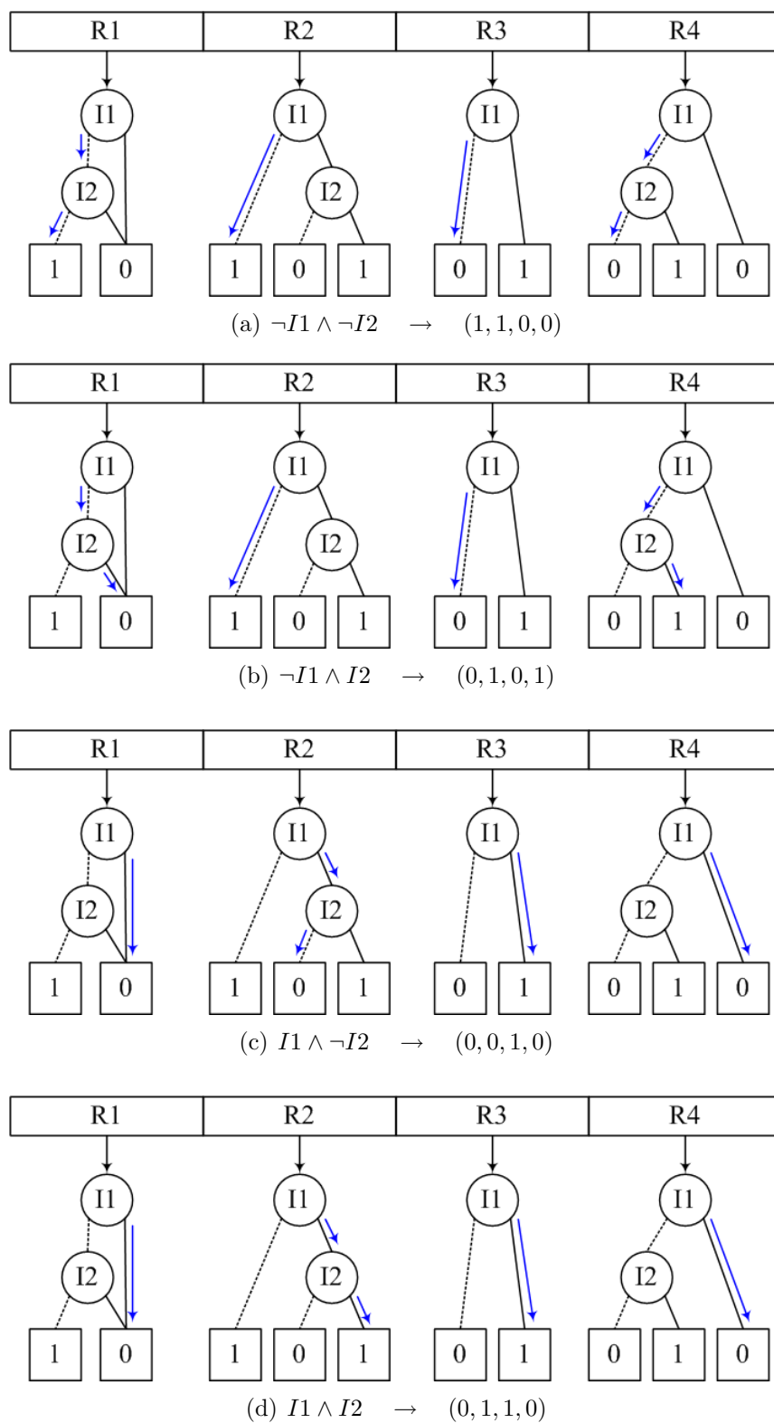
Figure 5.1: Analyse des vecteurs de BDDs des registres
