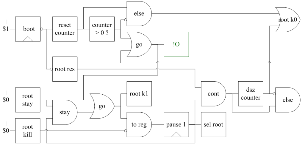
Figure 4.2: Le circuit du Programme 4.1 sans expansion des compteurs
