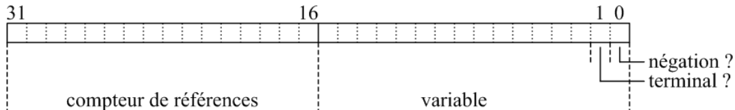
Figure 3.9: Têtes de nœuds de BDDs
