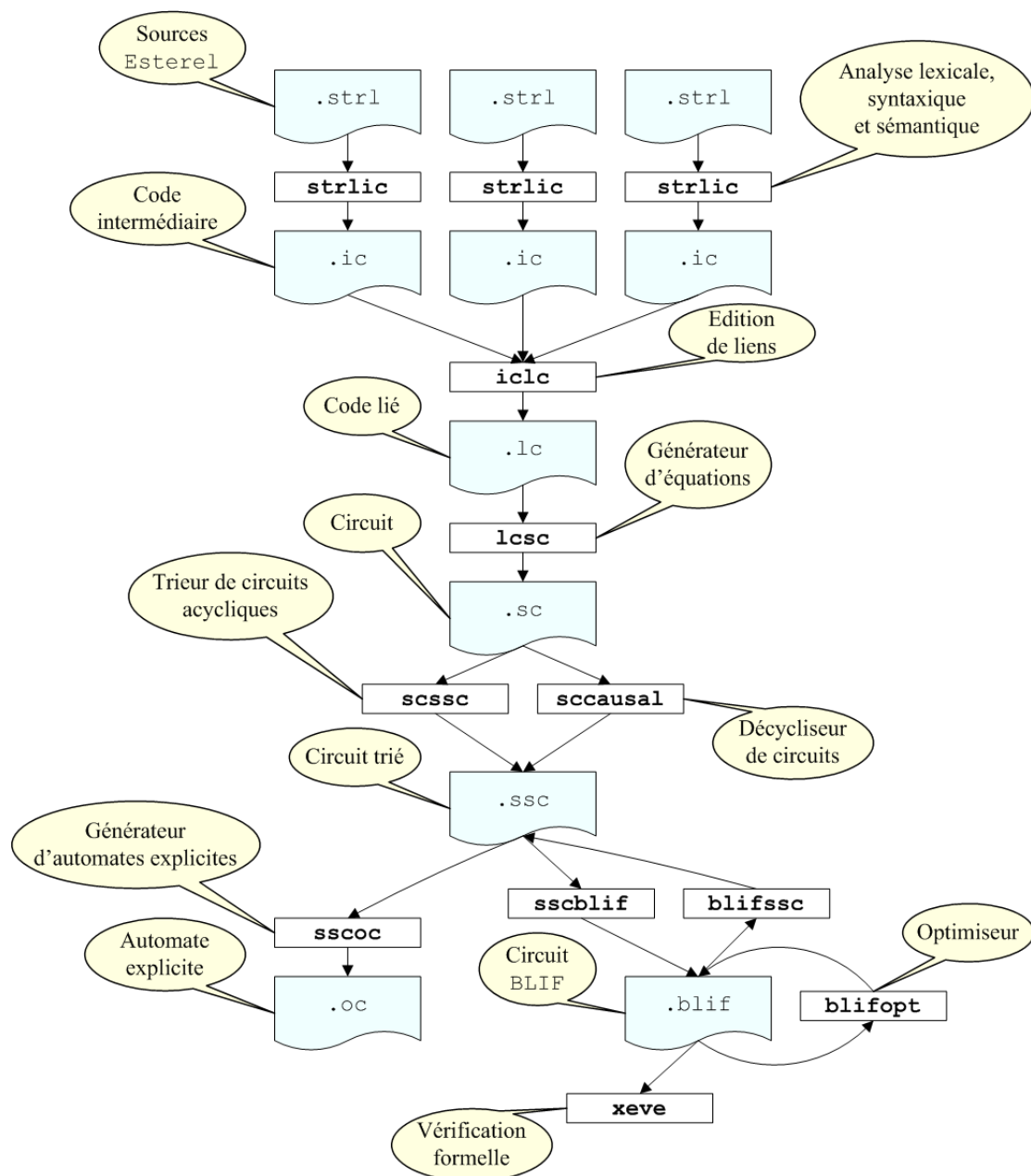
Figure 2.5: La chaîne de compilation d'Esterel v5_21
